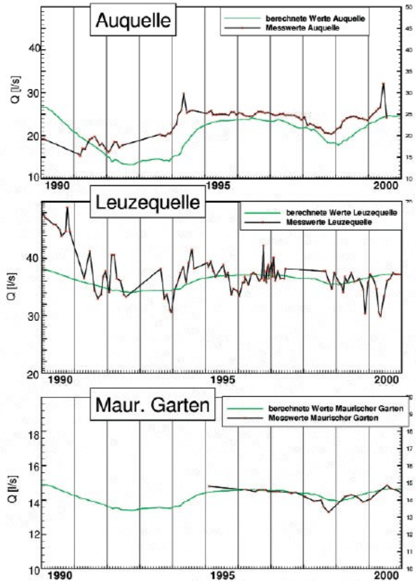
Abb. 5.16: Berechnete und gemessene Ganglinien an den Mineralquellen: Auquelle, Leuzequelle und Quelle im Maurischen Garten.
