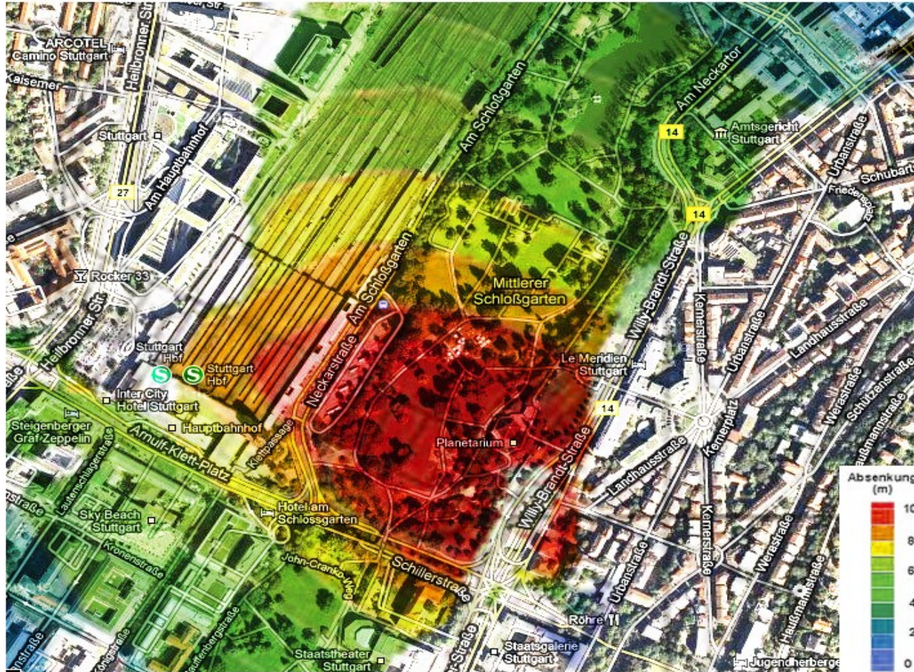
Grundwasserabsenkung ohne Infiltration: Weitreichender Absenktrichter gefährdet umliegende Bebauung. Simulation nach Kobus und Partner
