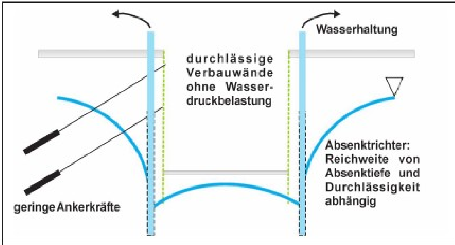
Abb. 1: Offene Wasserhaltung
