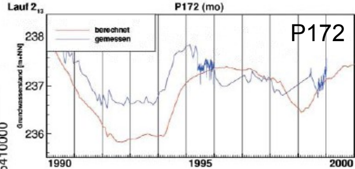
Abb. 5.15: Berechnete und gemessene Ganglinien an den Grundwassermessstellen P172, P174, P177 im Muschelkalkaquifer des Stuttgarter Talkessels.
