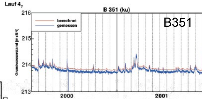
Abb. 5.19: Berechnete und gemessene Ganglinien an den Grundwasser- messstellen B351, B224 und am Sarweybrunnen jeweils im Unterkeuper zwischen 2000 und 2001.
